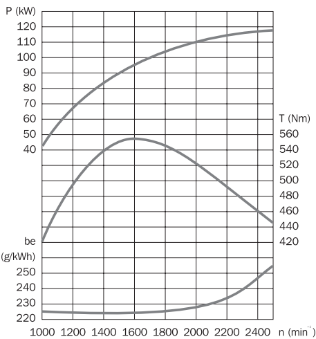
➔ BF6L 913
