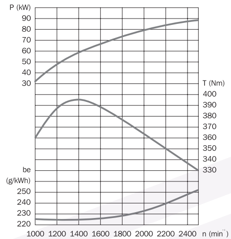
➔ F6L 913
